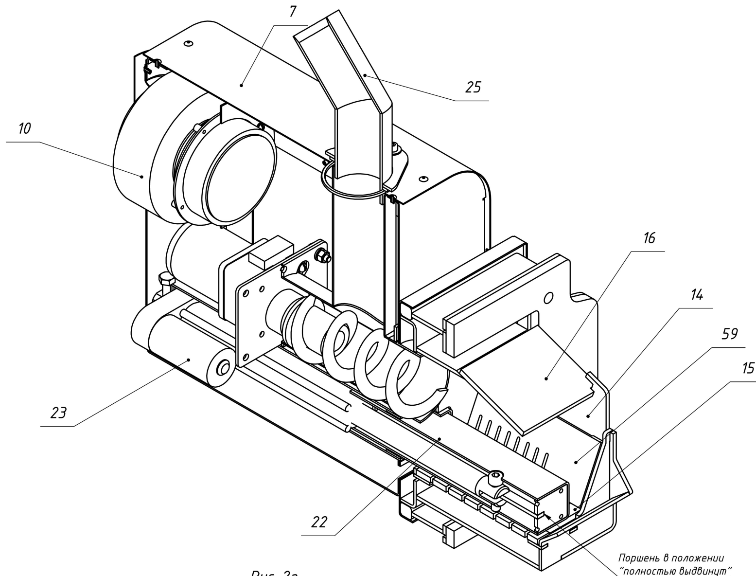
Рис. 2г Горелка пеллетная BC 4/35E (BC 10/50E).
