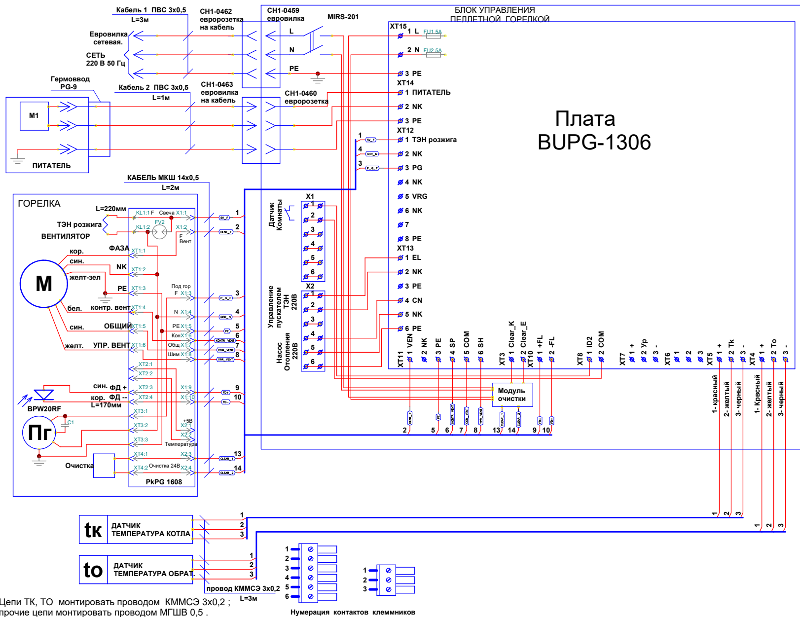
Рис. 8. Схема монтажная.
